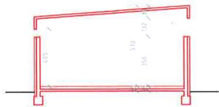
PRESJEK 1
