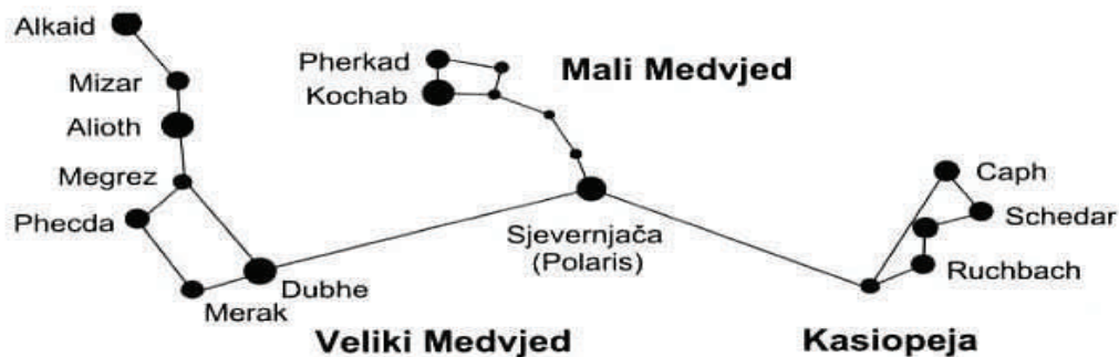
Slika 1. Položaj Sjevernjače
